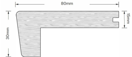
Bull nose edge soild
