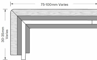
Flush mitre
