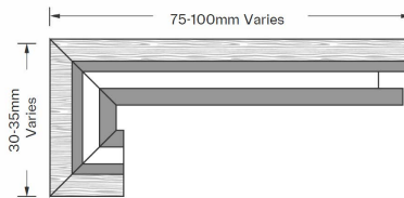
Overhung return mitre
